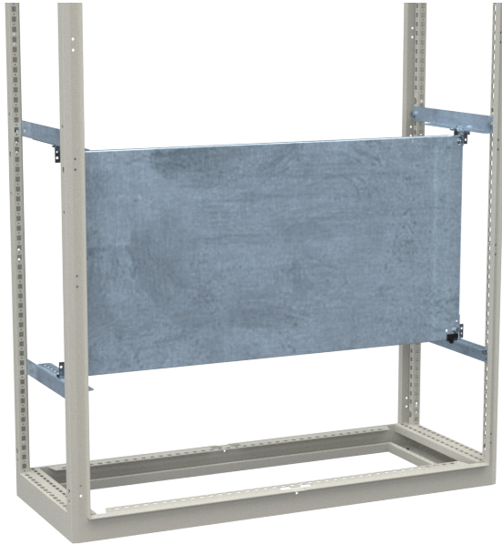
a) Montage auf mittlere Tragebügel siehe Seite 2
