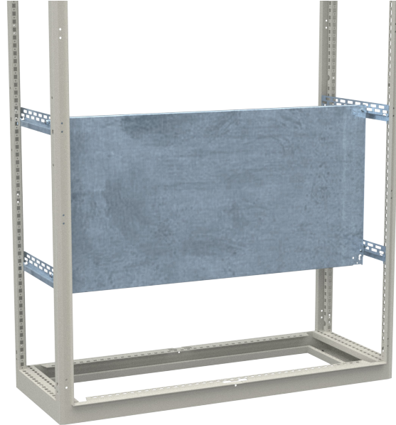
b) Montage an Mittenbefestigungen siehe Seite 3
